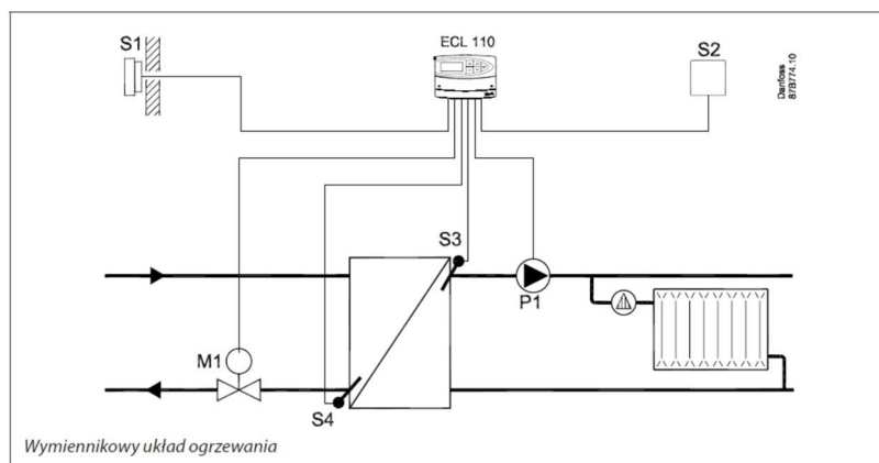
Rys. 26 a. Układ regulacji temperatury wody na zasilaniu instalacji c.o. w funkcji temperatury powietrza zewnętrznego (tzw. regulacja „pogodowa”) (Źródło: www.danfoss.pl )
