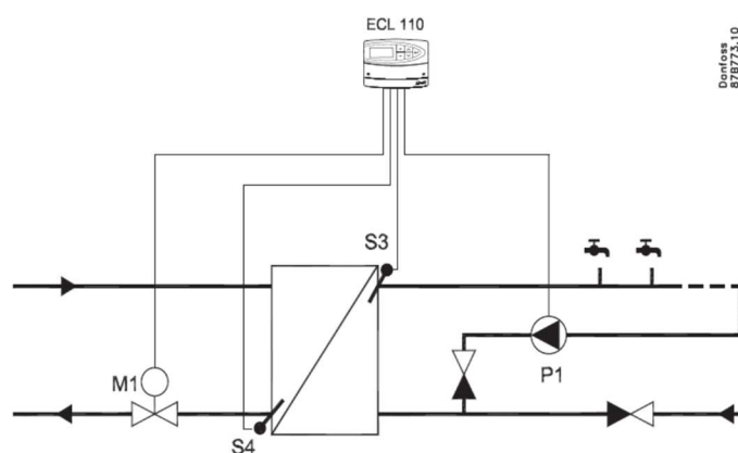
Rys. 26 b. Układ regulacji temperatury wody na zasilaniu instalacji c.w.u. (Źródło: www.danfoss.pl )
