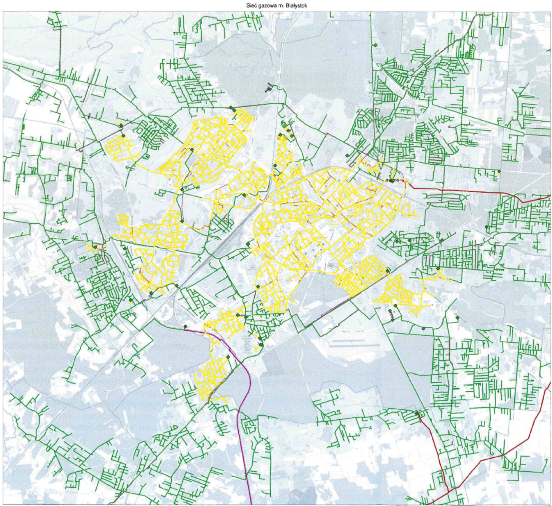
Rys. 22. Układ istniejących sieci gazowych na terenie Białegostoku
