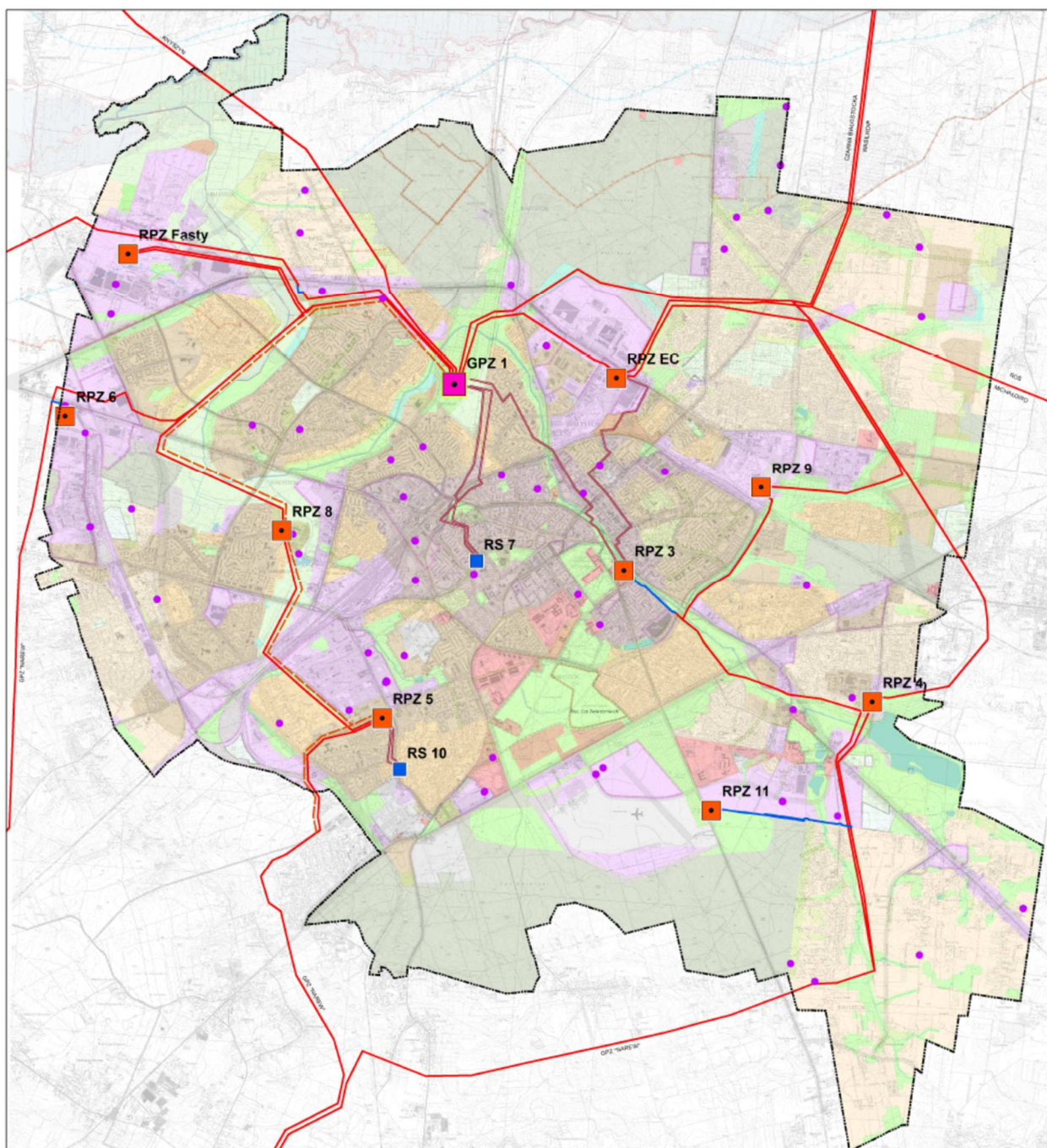
Rys. 23. Układ zasilania sytemu elektroenergetycznego na terenie Białegostoku (Źródło: „Studium uwarunkowań i kierunków zagospodarowania przestrzennego miasta Białegostoku” Białystok 2019, 2023)
