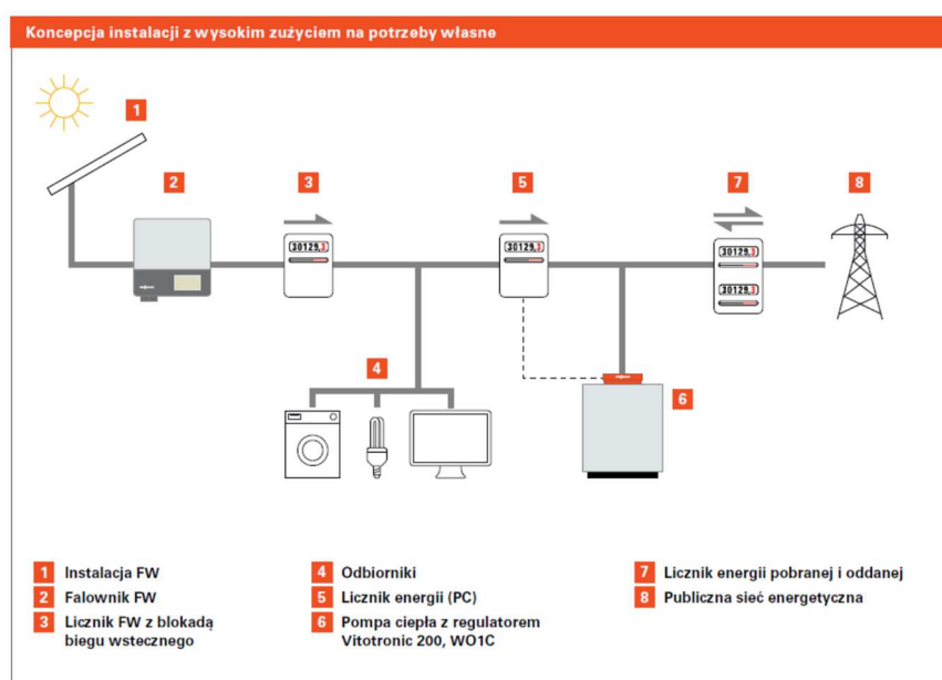
Rys. 31. Schemat domowej instalacji fotowoltaicznej (Źródło: www.viessmann.pl )
