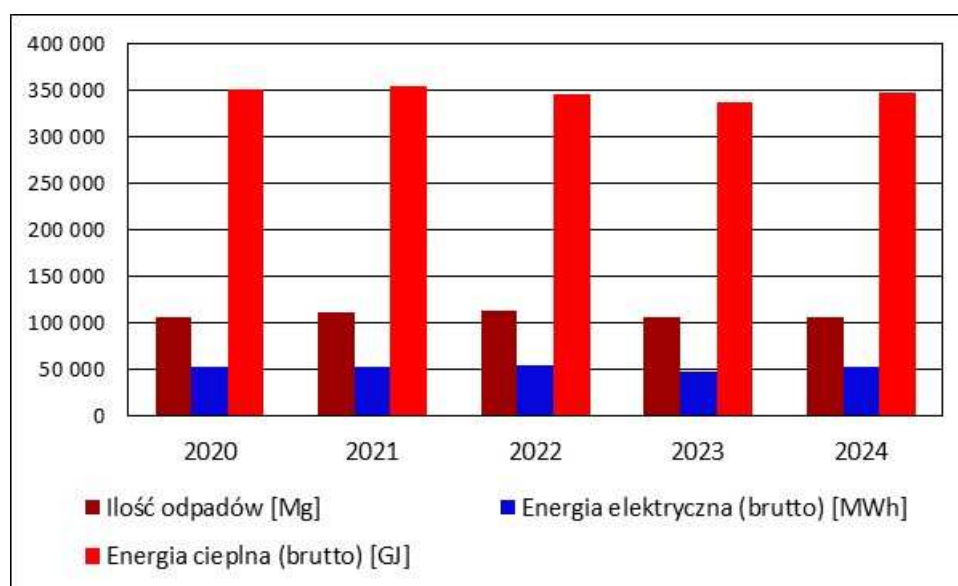
Rys. 8. Wykorzystanie odpadów oraz produkcja energii elektrycznej i ciepłej w ZUOK w latach 2020 - 2024
