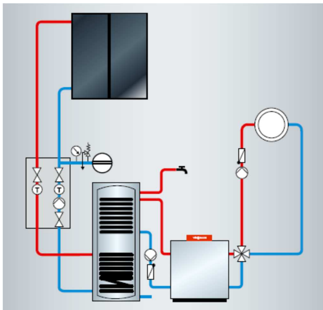
Rys. 32. Układ technologiczny wykorzystania energii promieniowania słonecznego do podgrzewu ciepłej wody użytkowej (Źródło: www.viessmann.pl )
