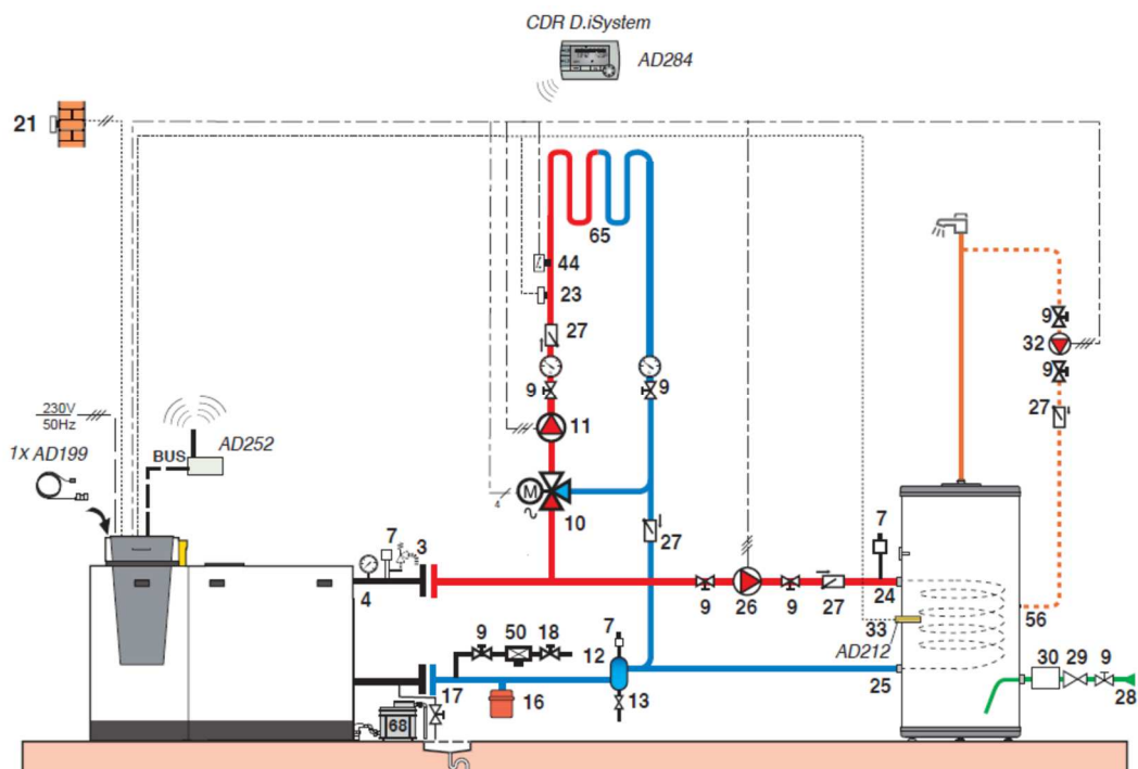
Rys. 28. Schemat kotłowni opalanej paliwem ciekłym lub gazowym (Źródło: www.dedietrich.pl )
