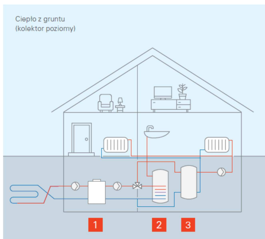
Rys. 34. Układ pompy ciepła z poziomym wymiennikiem gruntowym 1 –pompa ciepła, 2 – podgrzewacz c.w.u., 3 – zbiornik buforowy (Źródło: www.viessmann.pl )
