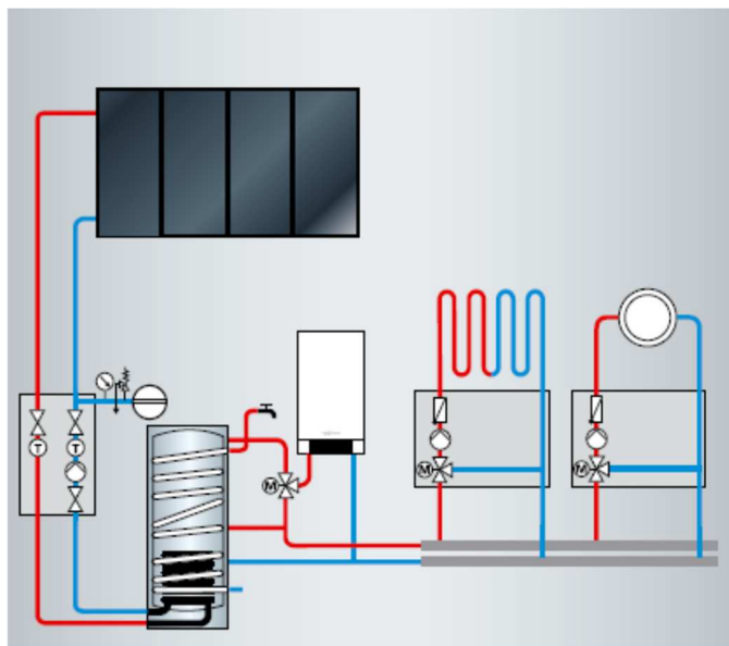
Rys. 33. Układ technologiczny wykorzystania energii promieniowania słonecznego do podgrzewu ciepłej wody użytkowej oraz w pracy instalacji centralnego ogrzewania (Źródło: www.viessmann.pl )
