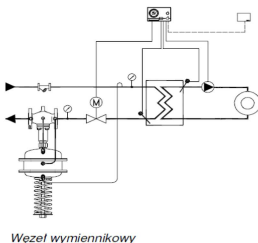
Rys. 26 c. Układ regulacji różnicy ciśnień z ograniczeniem maksymalnego przepływu wody sieciowej przez węzeł (Źródło: www.danfoss.pl )
