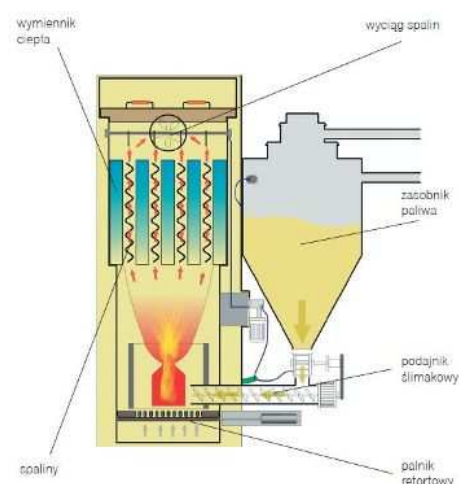
Rys. 39. Widok i przekrój kotła do spalania zrębków lub peletów drewnnych (Źródło: www.termomodernizacja.pl )
