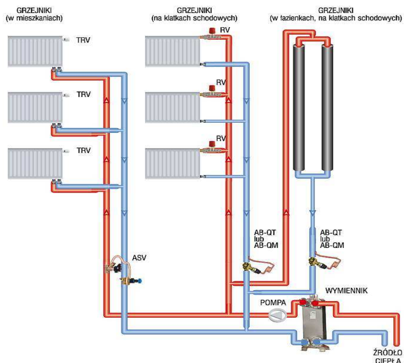
Rys. 25. Schemat instalacji centralnego ogrzewania z zalecanymi układami automatycznej regulacji: TRV – zawory regulacyjne z nastawami wstępnymi i z głowicami termostatycznymi, RV - zawory regulacyjne z nastawami wstępnymi, AB-QT lub AB-QM – zawory regulacyjne natężenia przepływu z ograniczeniem maksymalnej temperatury (QT) lub ograniczeniem maksymalnego przepływu (QM)
